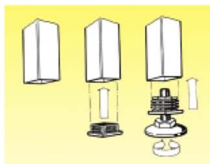
Стандартная ножка. В центре. Нивелирная ножка. Справа. (на заказ) Оптимальный вариант для сглаживания небольших неровностей.
